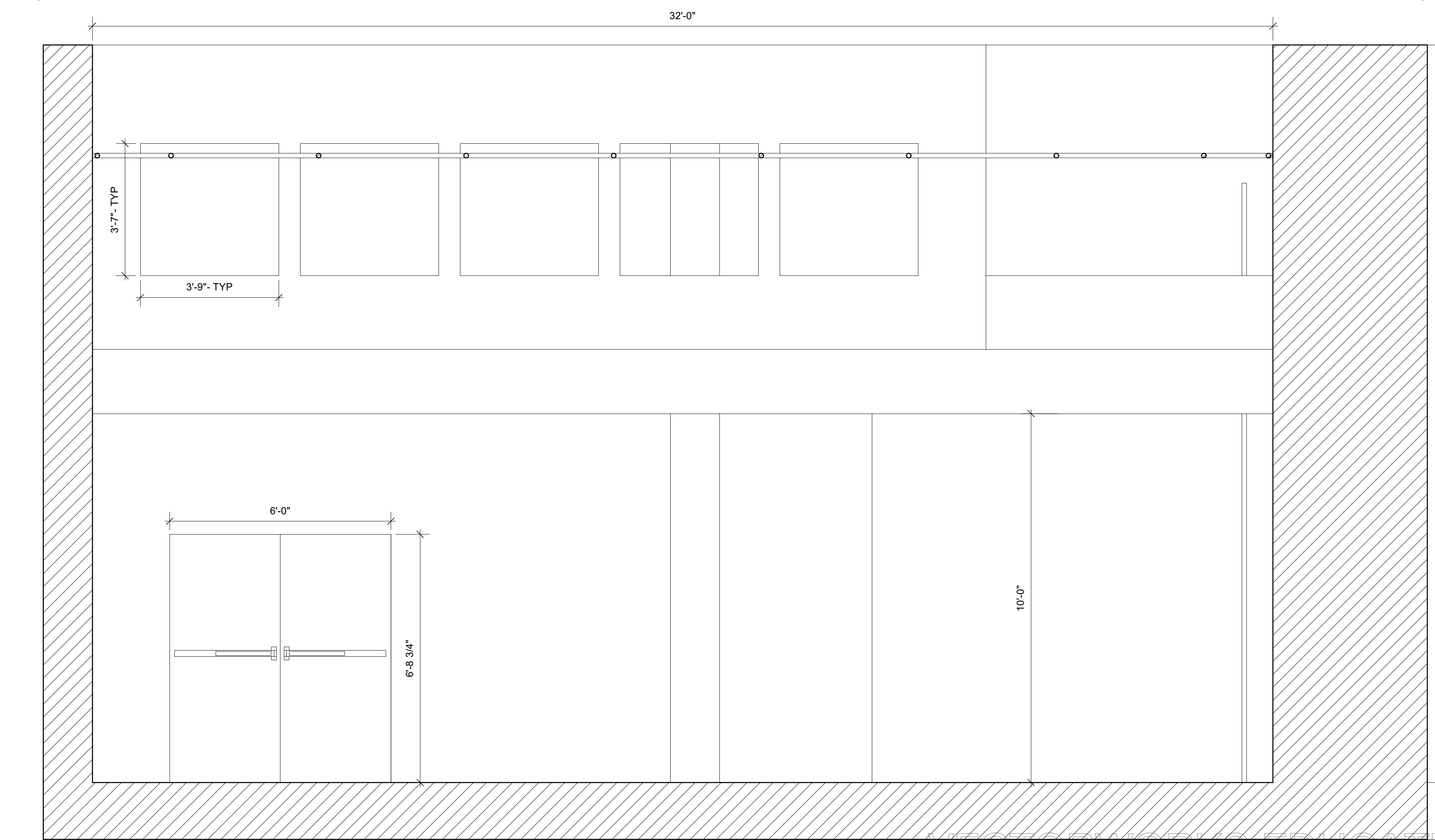
5 BOOTH WALL Scale: 1/2" = 1'-0"
