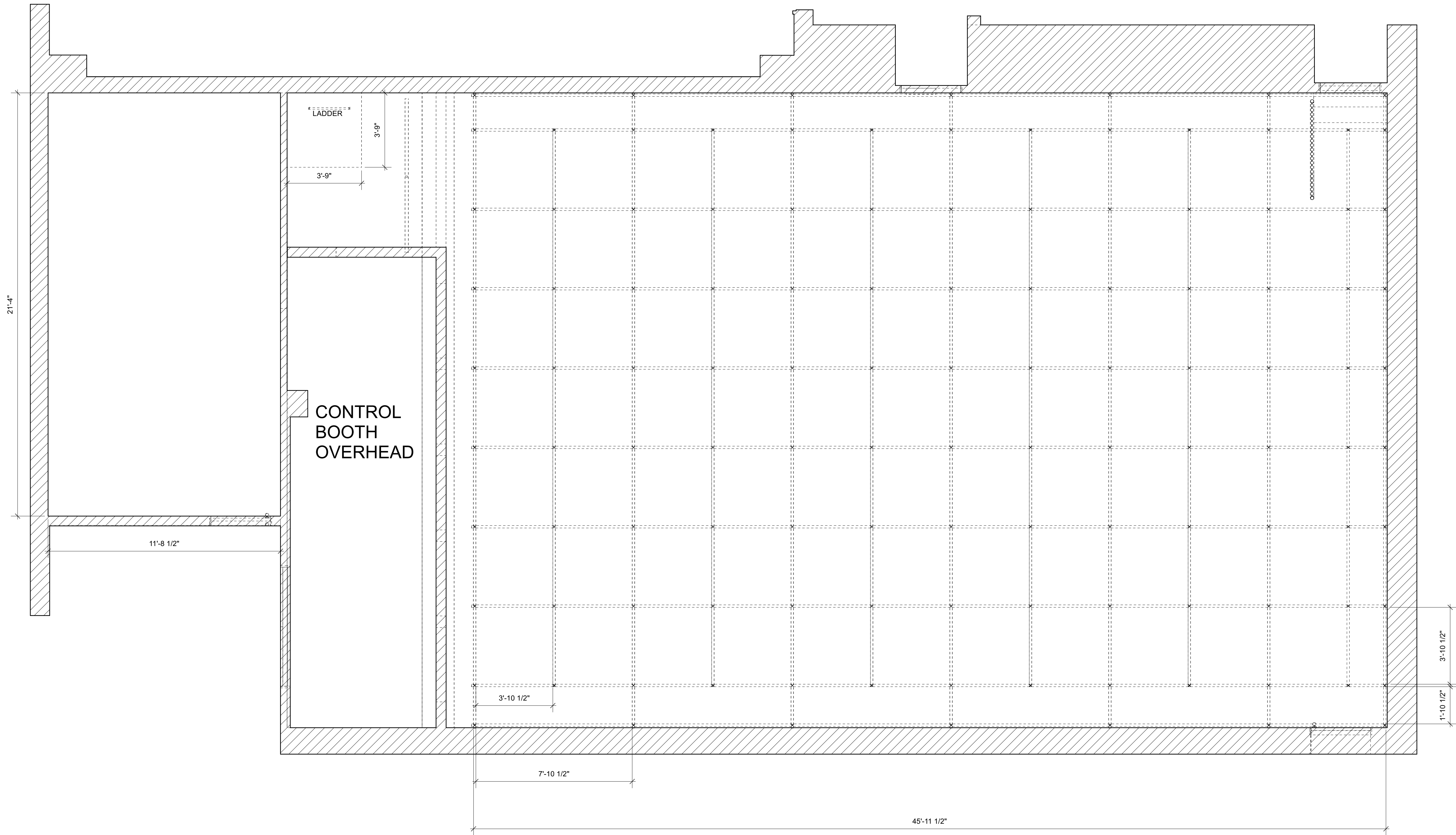
2 GRID LAYOUT Scale: 3/8" = 1'-0"
